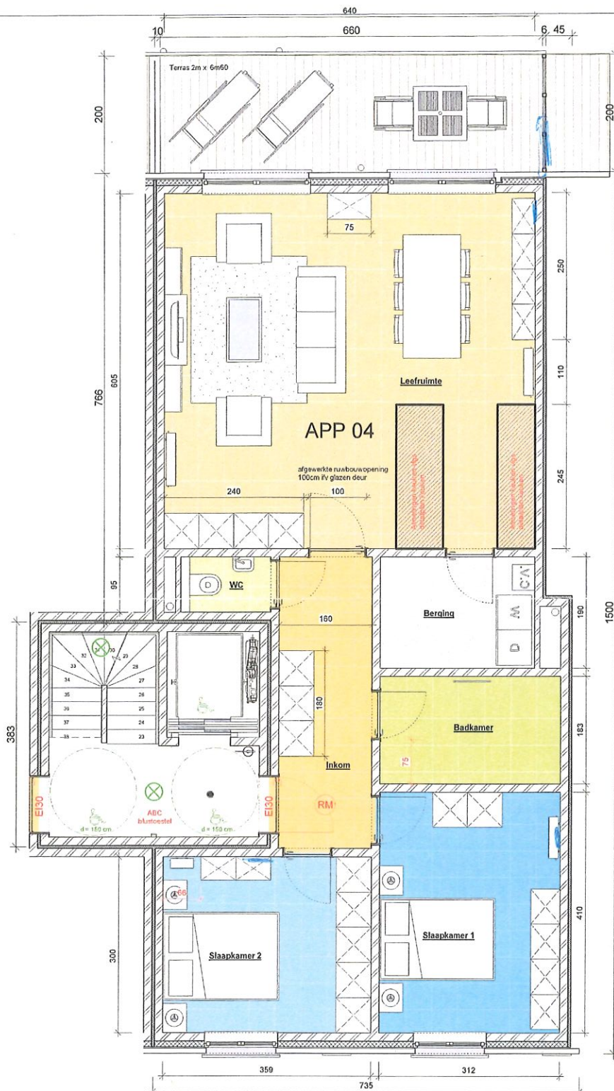
4 Appartement 04 1:50
