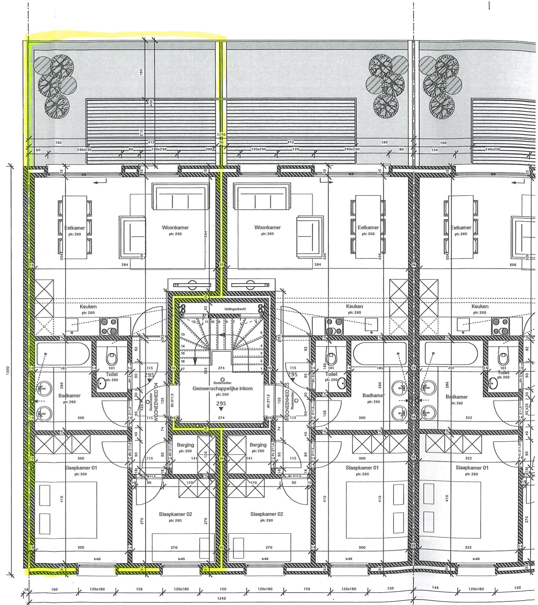
VERDIEPING 1 schaal 1/75
